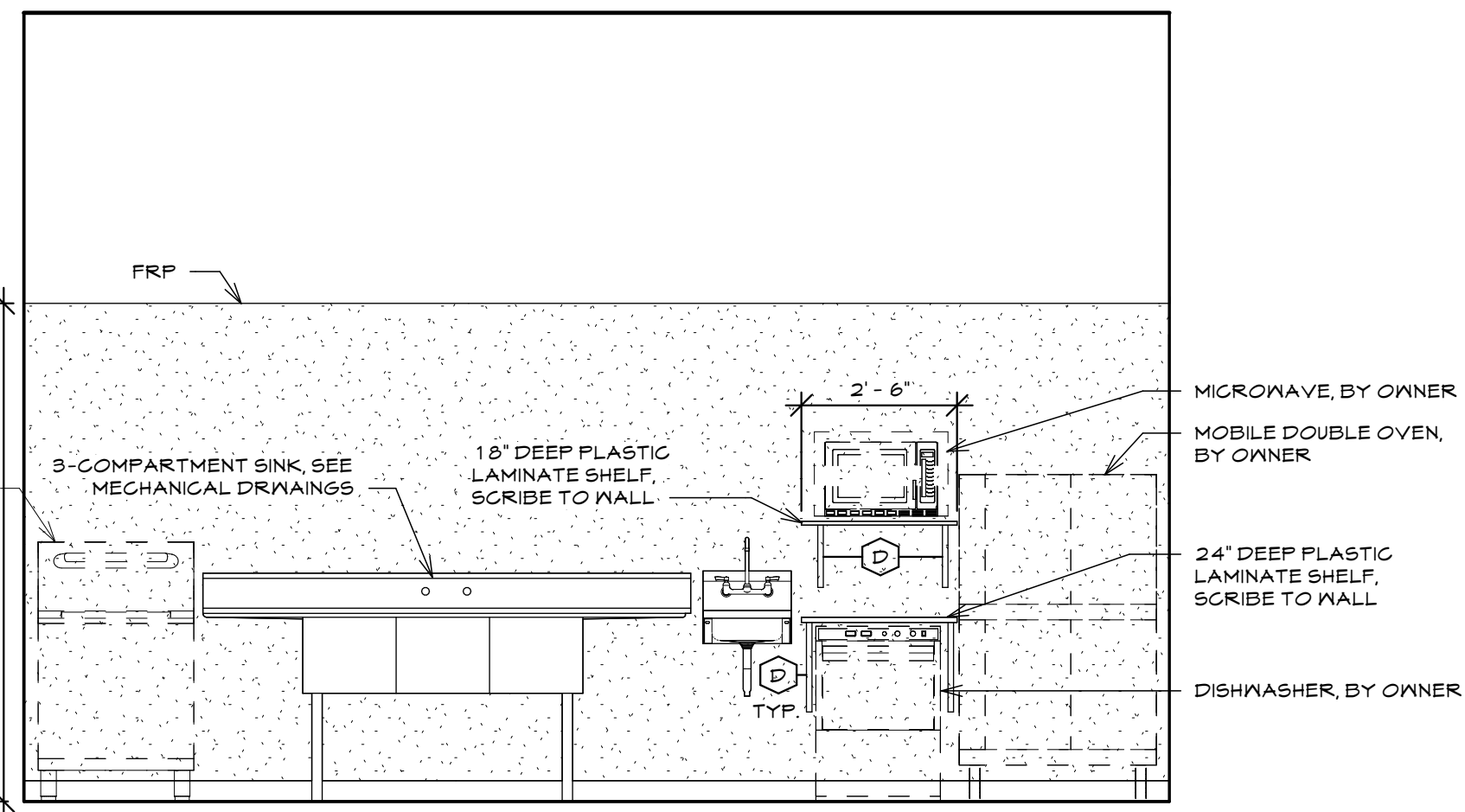
⑧ CATERING SCALE: 3/8" = 1'-0" ROOM 215
