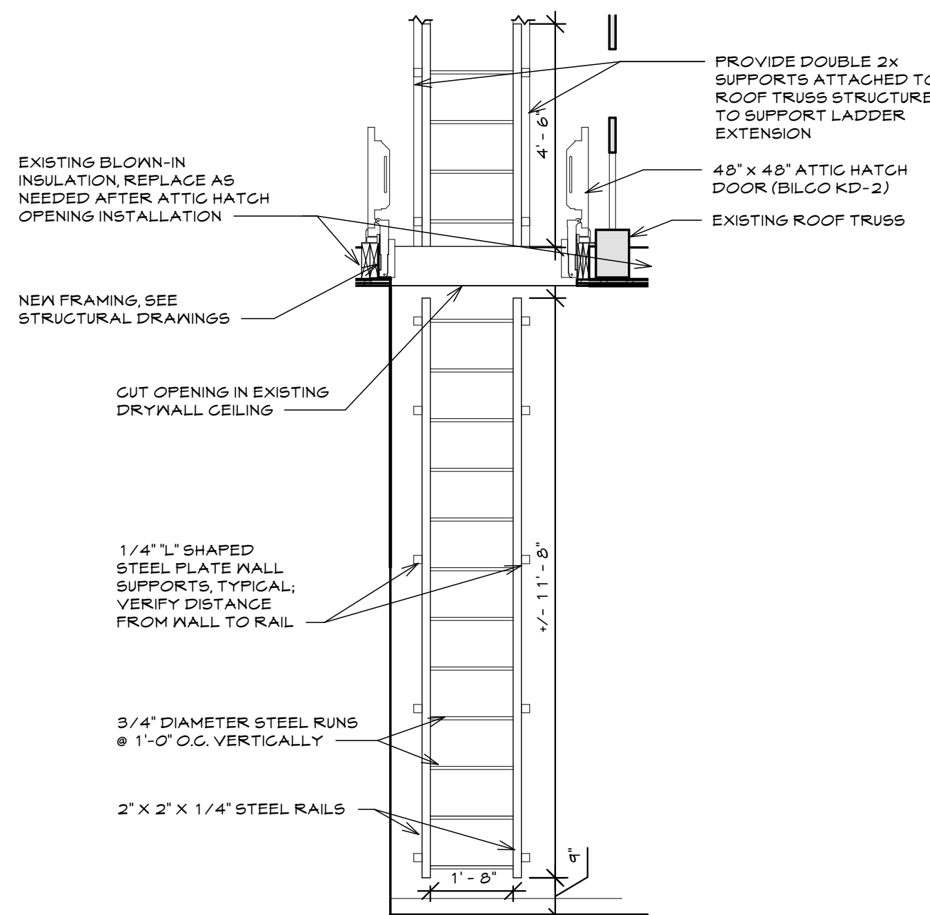
㉑ LADDER SCALE: 3/8" = 1'-0"
