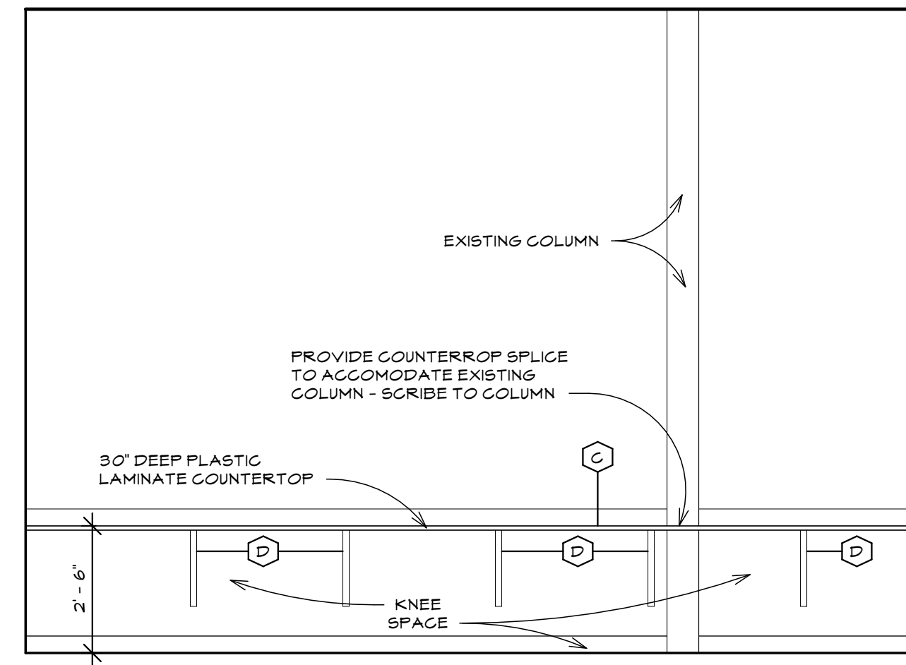
⑲ OFFICE SCALE: 3/8" = 1'-0" ROOM 202
