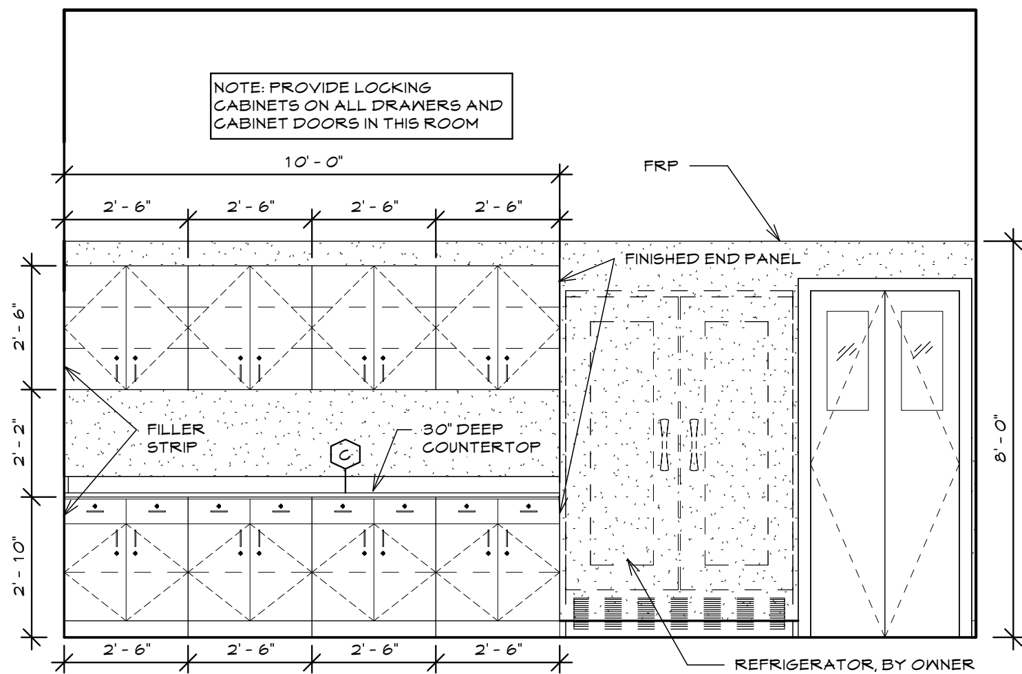
⑦ CATERING SCALE: 3/8" = 1'-0" ROOM 215
